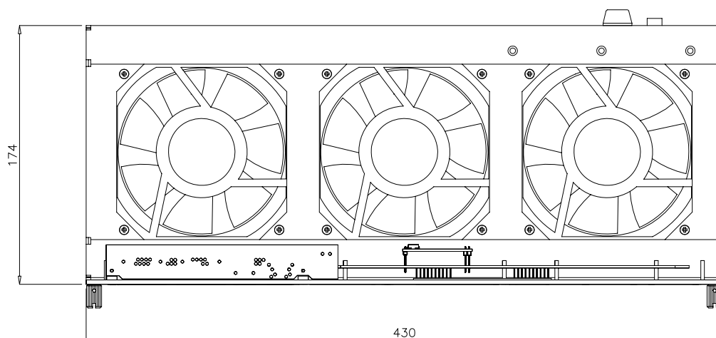
Fig. 2.8: Mod A8160 Smart VME Fan Unit Top view
